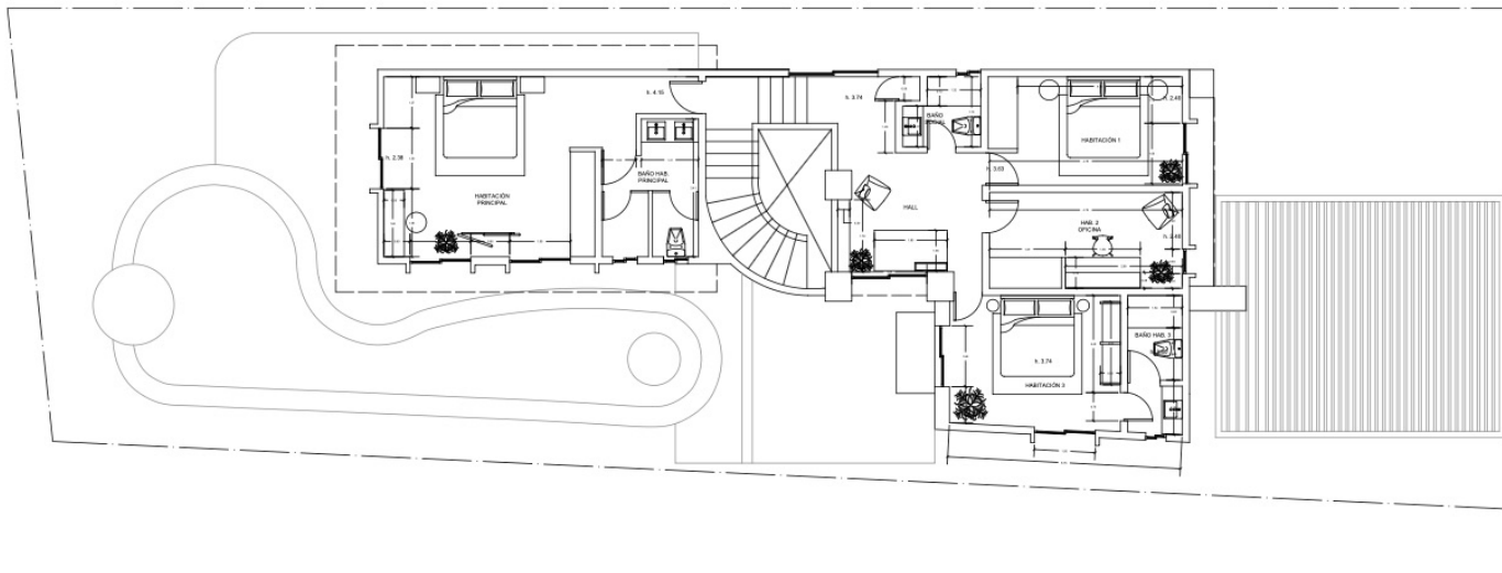
PLANTA ALTA
